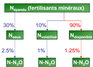
Figure 5. Exemple de schéma de calcul des émissions de N 2 O dans la méthode actuelle du CITEPA (GIEC 1996).
